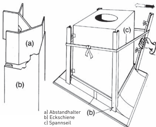
Eckschiene im Profil
